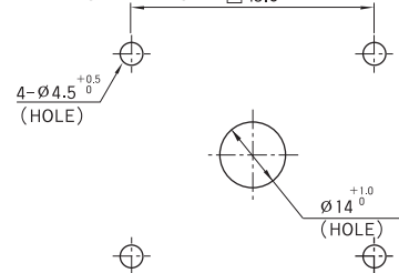
開孔尺寸 (60×60)
